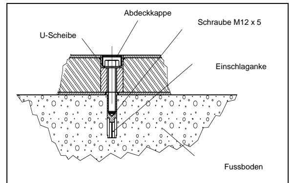
Skizze der Bodenbefestigung
